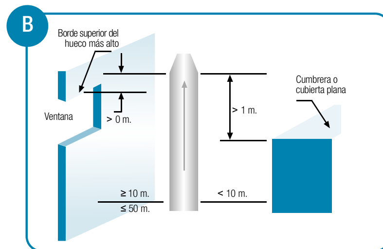
Chimeneas construidas entre dos obstáculos
