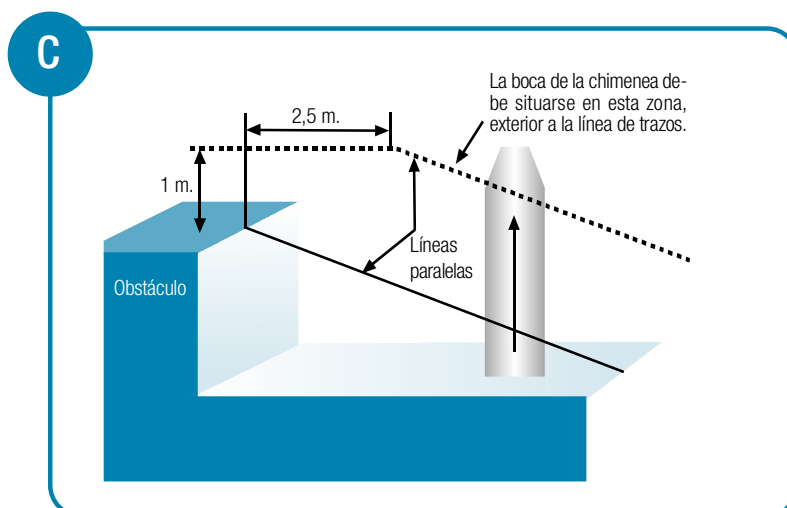
Chimeneas construidas sobre cubiertas planas
