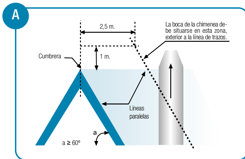
Chimeneas construidas sobre cubiertas inclinadas
